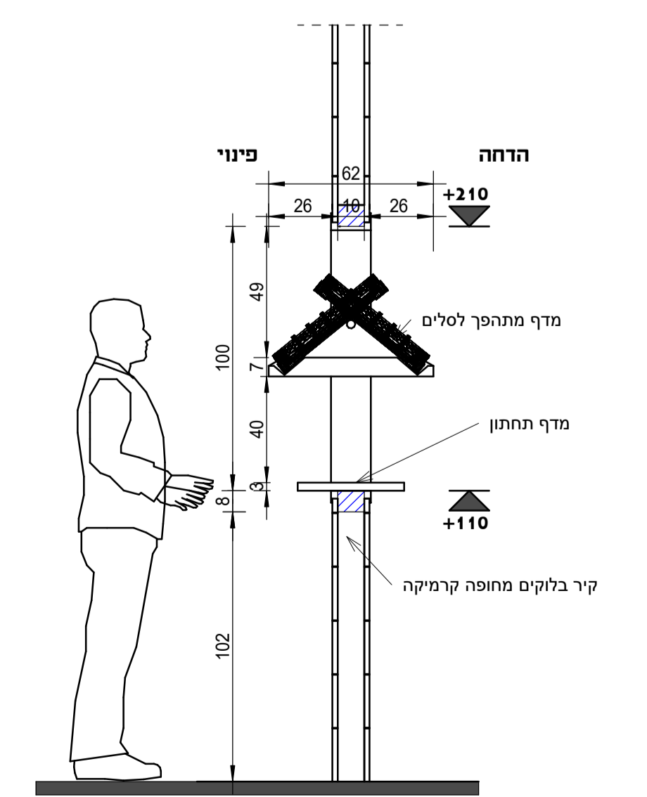
חיתת אשנב הוצאת מנות קב"מ 1:20
