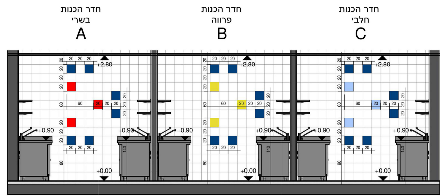
פריסת קיר בחדרי ההכנת קב"מ 1:50
