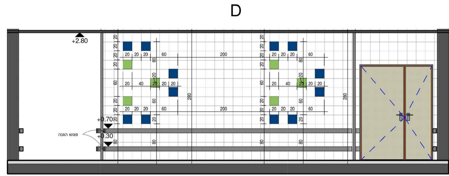
פריסת קיר במסדרון קב"מ 1:50
