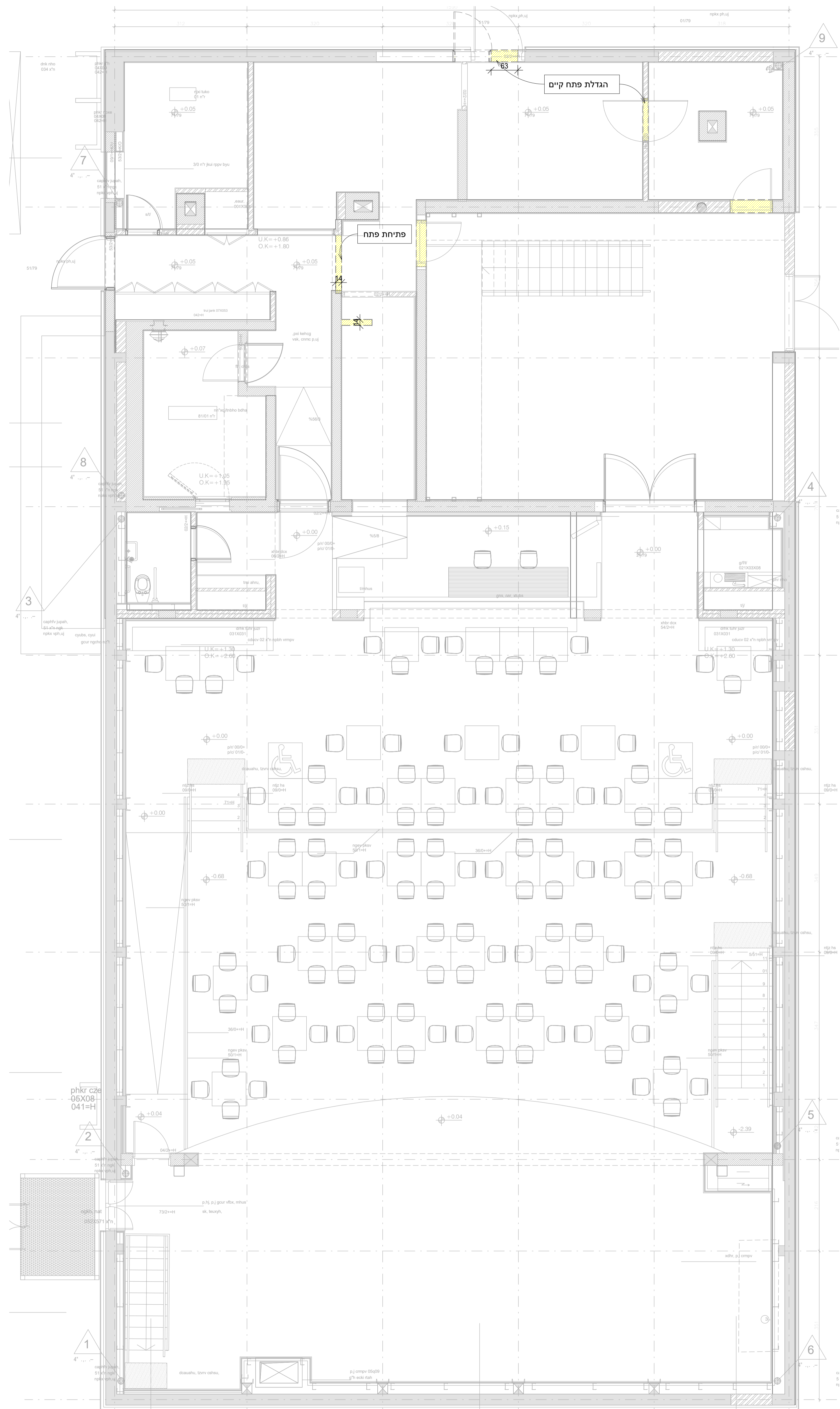
תוכנית הריסת קב"מ 1:50
