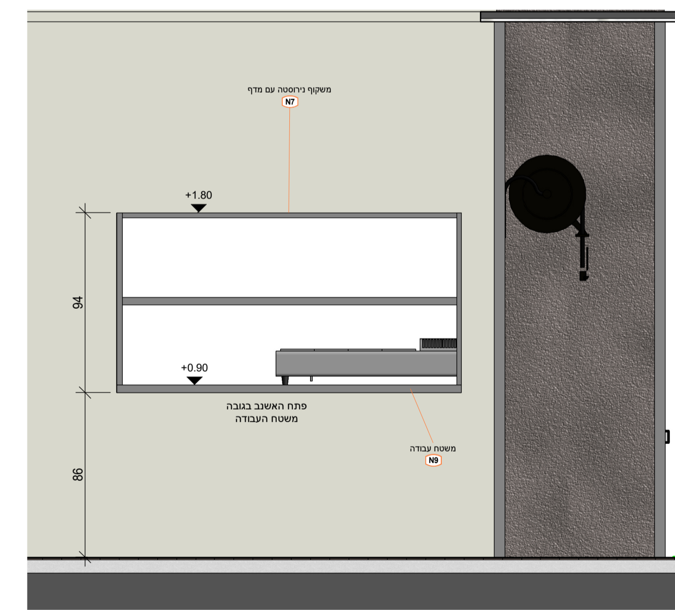
חיתת אשנב הוצאת מנות קב"מ 1:20
