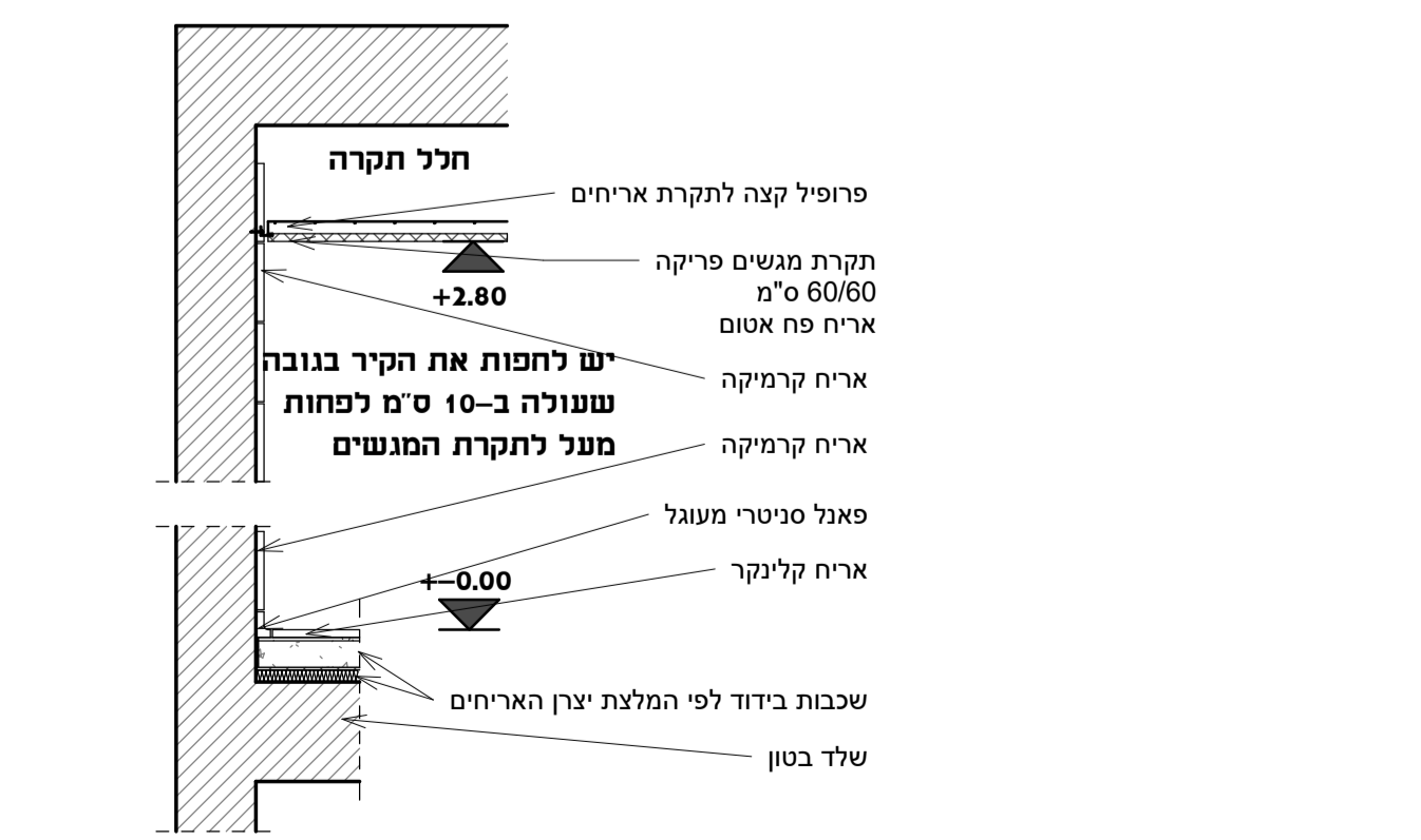
פריסת קיר במסדרון קב"מ 1:50
