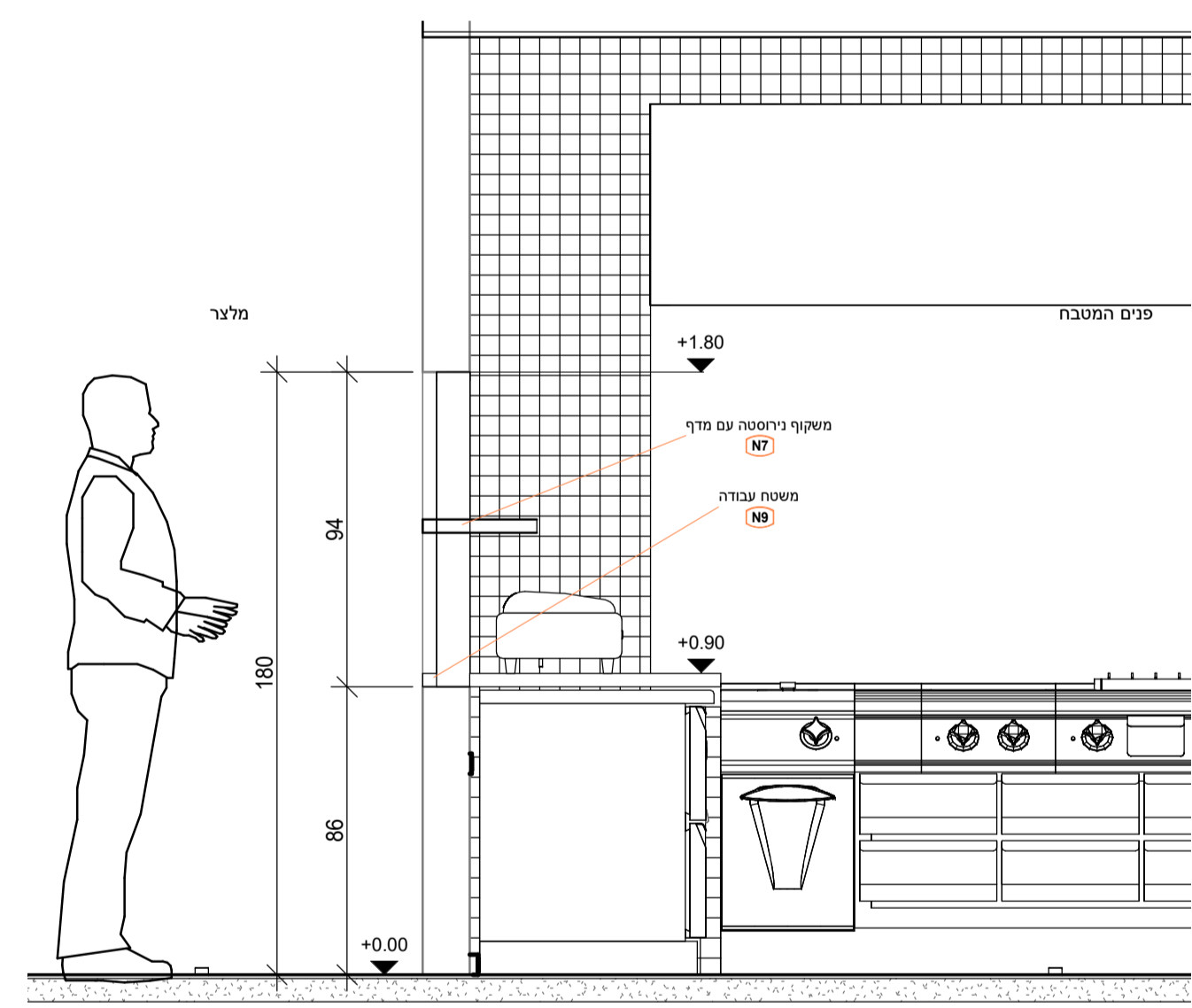
חיתת אשנב הוצאת מנות קב"מ 1:20
