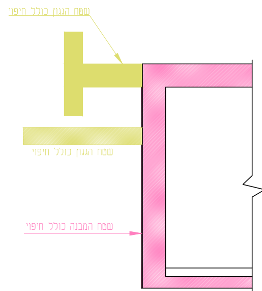
חתך שיפוסי לגגון כפול
