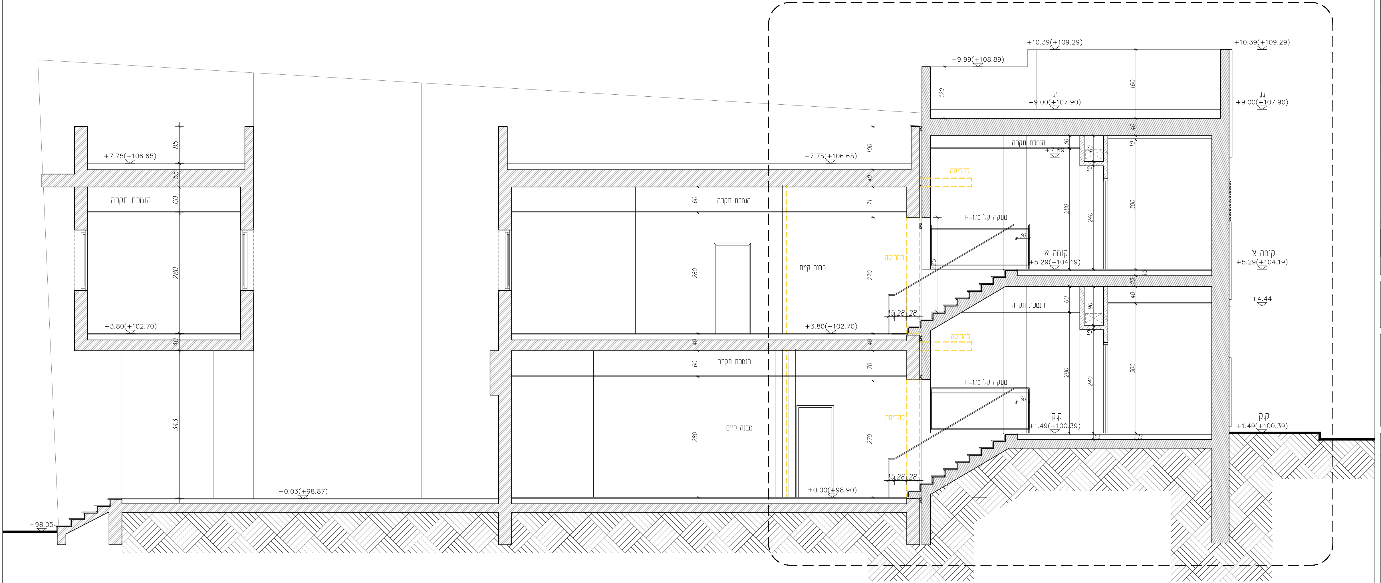
חֶתֶךְ N-N
