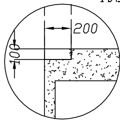
פרט רצפה ללא ריצוף
