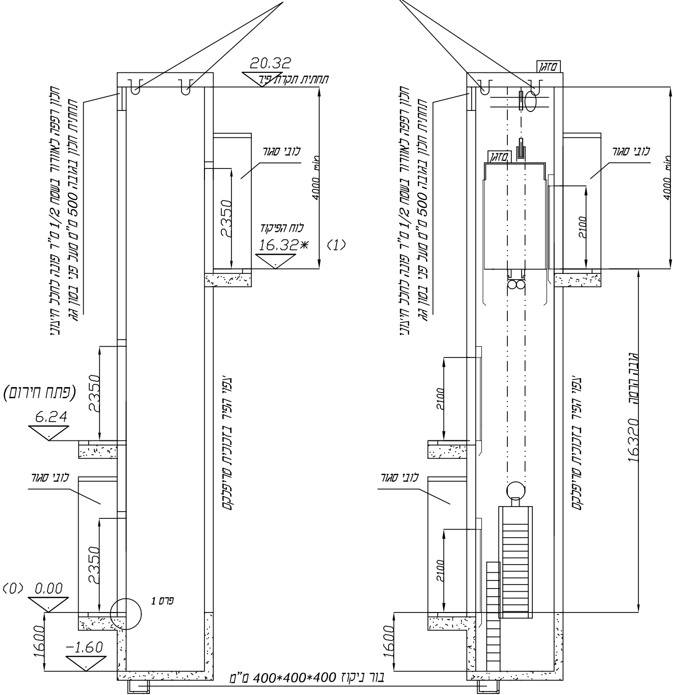
חתך 1-1 תכנית בניה
