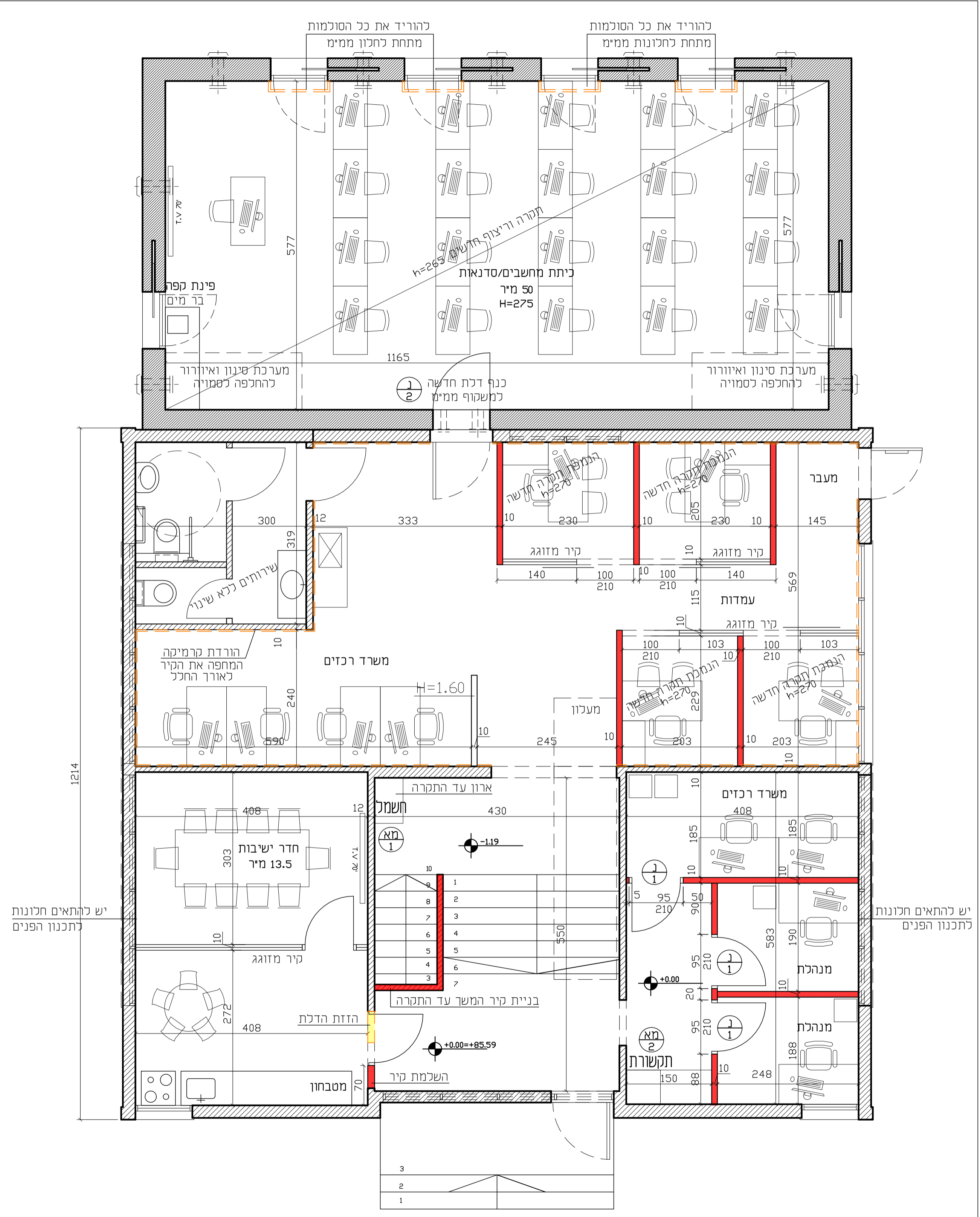
תכנית קומת קרקע קנ"מ 1:50 מצב מוצע
