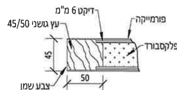
פרט בנף עץ 1:50
