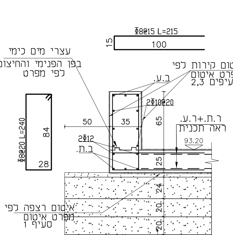
חתך 1-1 1:25
