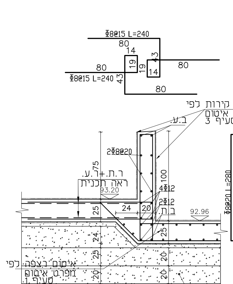
חתך 2-2 1:25
