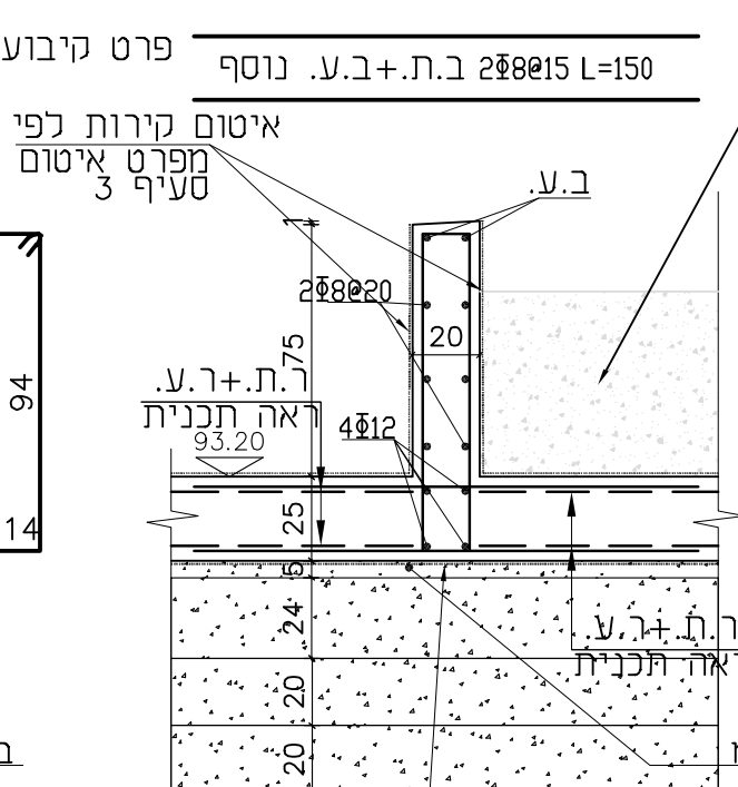
חתך 4-4 1:25
