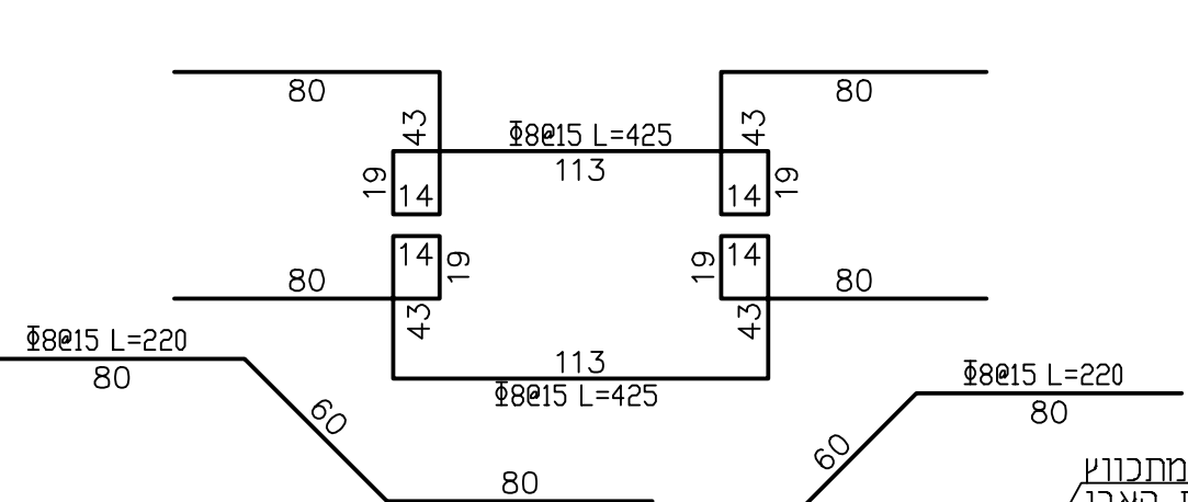
חתך 3-3 1:25
