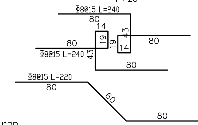
חתך 5-5 1:25
